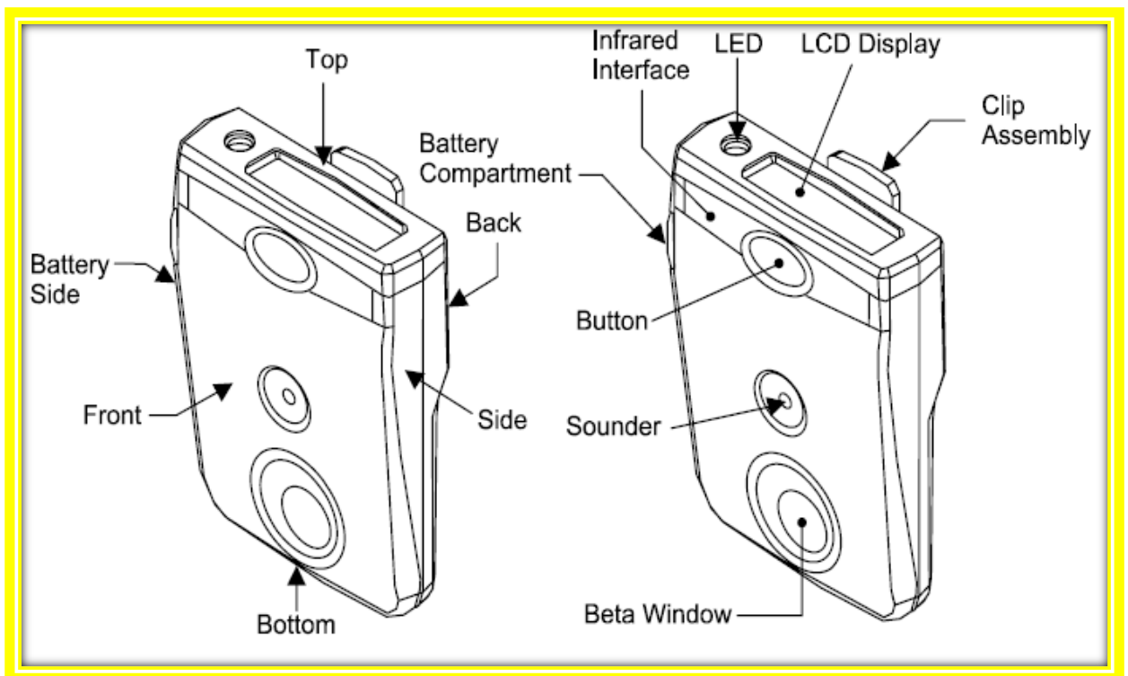
Slika 6. Elektronski dozimeter
