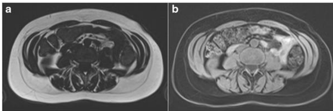
Slika 9 T1W transverzalne Dixon MR slike: a) prikaz signala masti b) prikaz signala vode u razini L3 kralješka
