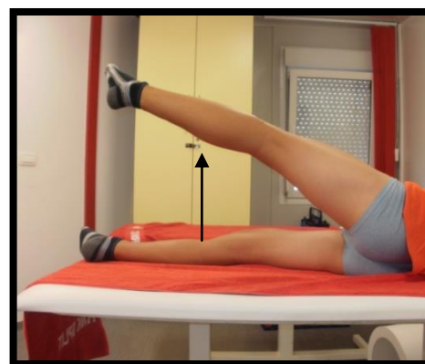
Slika 21. Abdukcija natkoljenice
