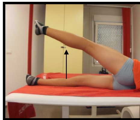
Slika 21. Abdukcija natkoljenice
