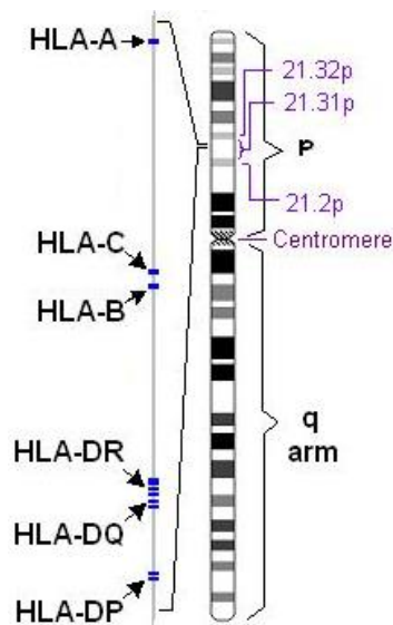
Slika 1. Šesti kromosom
