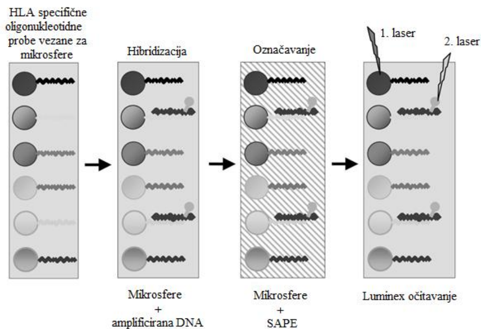
Slika 9. Princip PCR-SSO metode
