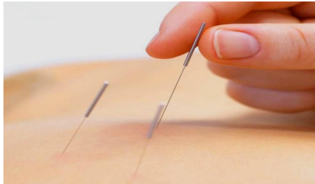
Slika 15. Akupunktura
